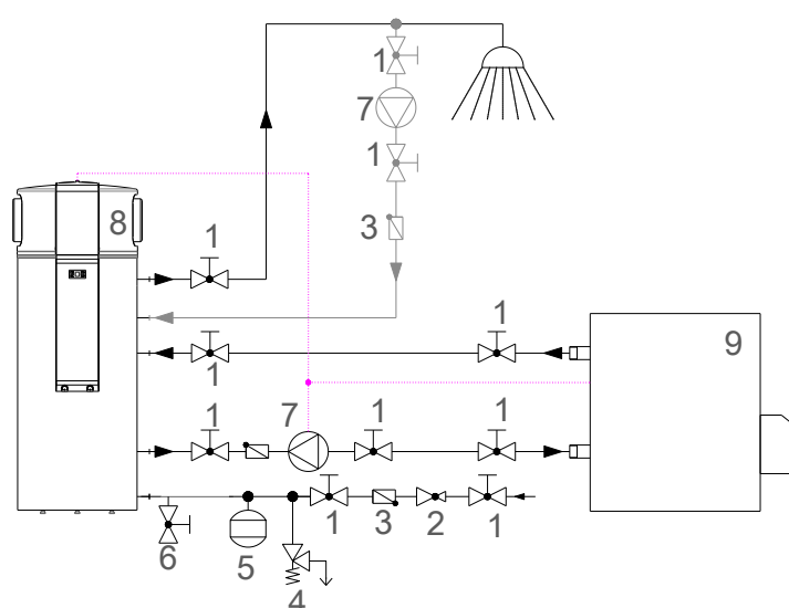
Afbeelding 3: Warmtepomp in combinatie met ketel
