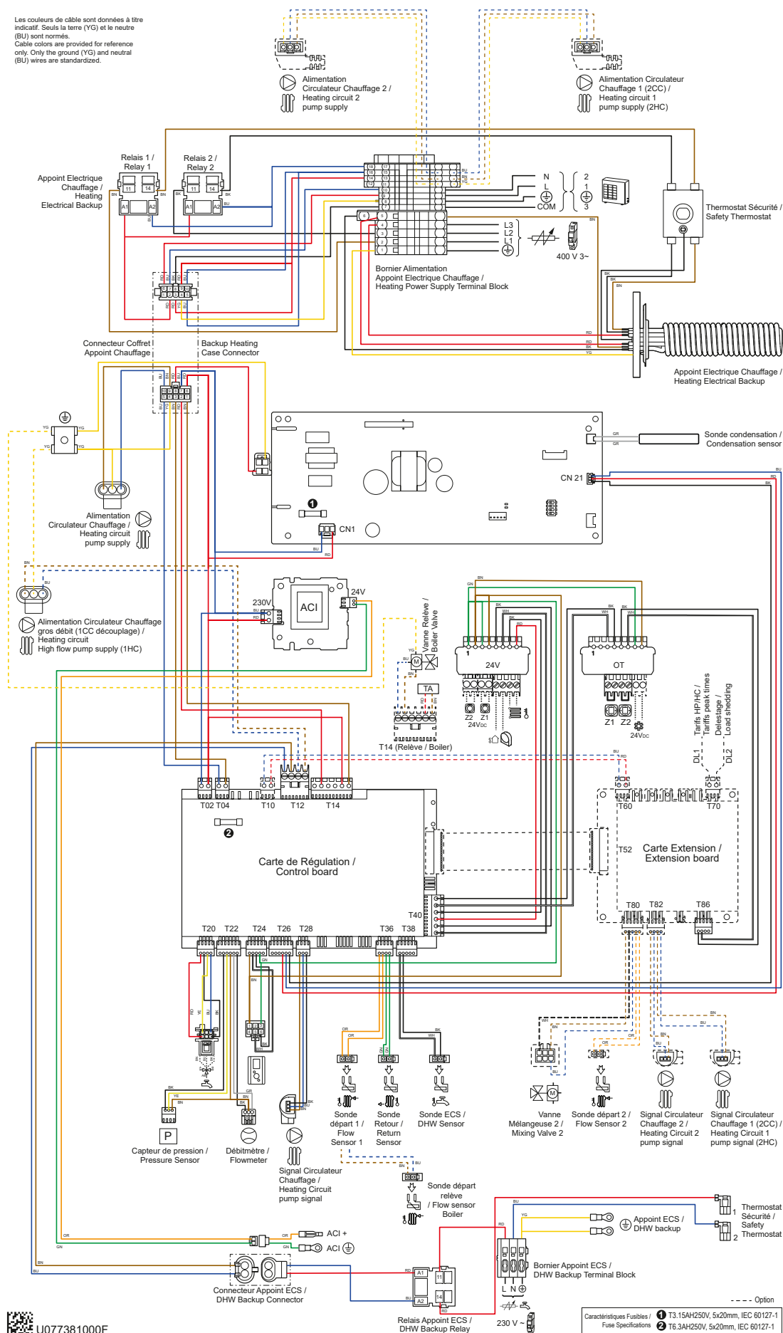
fig. 47 - Elektrische kablering hydraulische module - driefasig model
