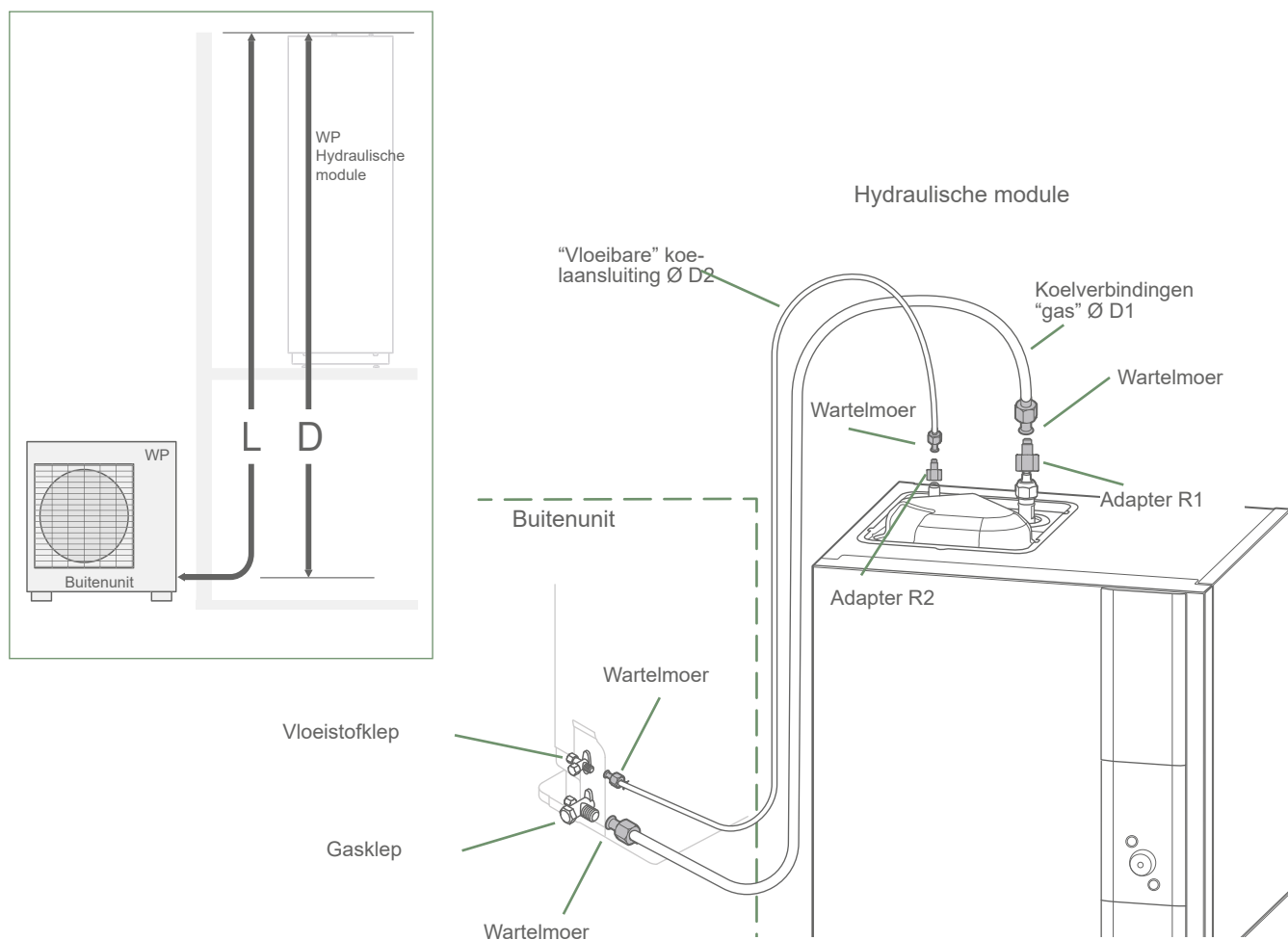
fig. 31 - Aansluiting van koelverbindingen (toegestane diameters en lengtes)
