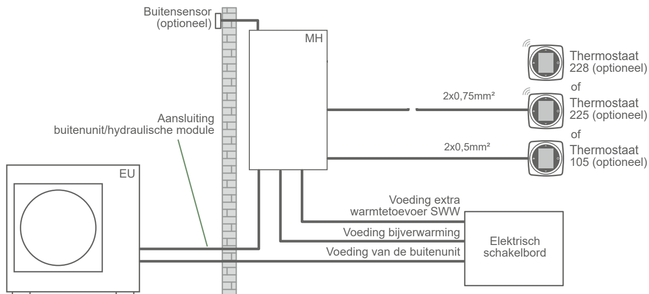
fig. 37 - Overzicht van elektrische aansluitingen voor eenvoudige installatie (1 verwarmingskring)
