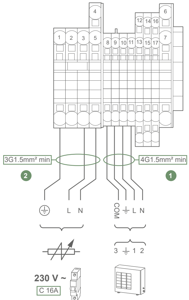
fig. 12 - Aansluitingen Voeding
