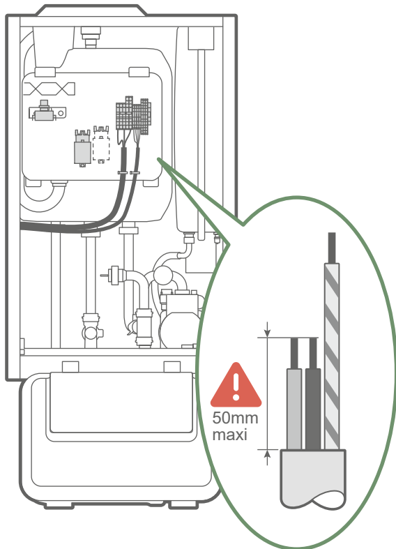
fig. 13 - Kabeldoorgangen
