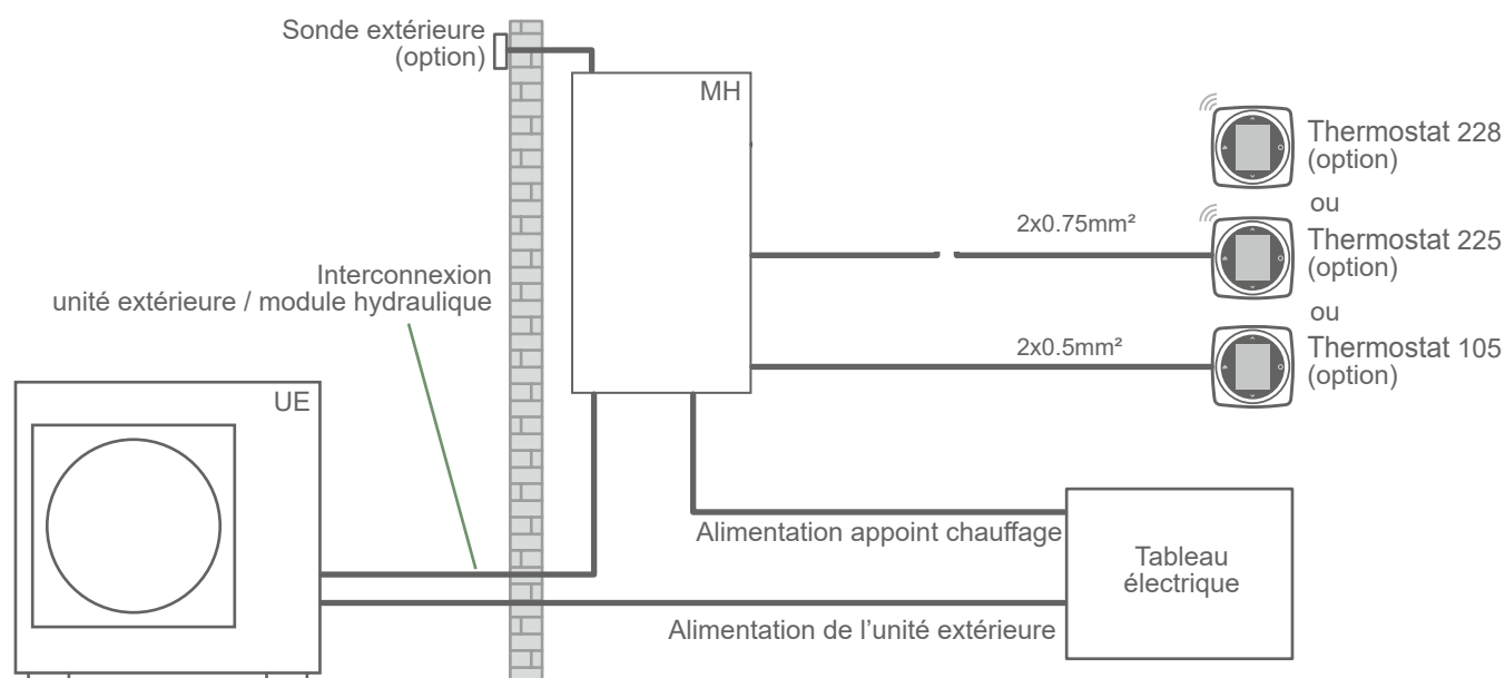
fig. 37 - Schéma d'ensemble des raccordements électriques pour une installation simple (1 circuit de chauffe)
