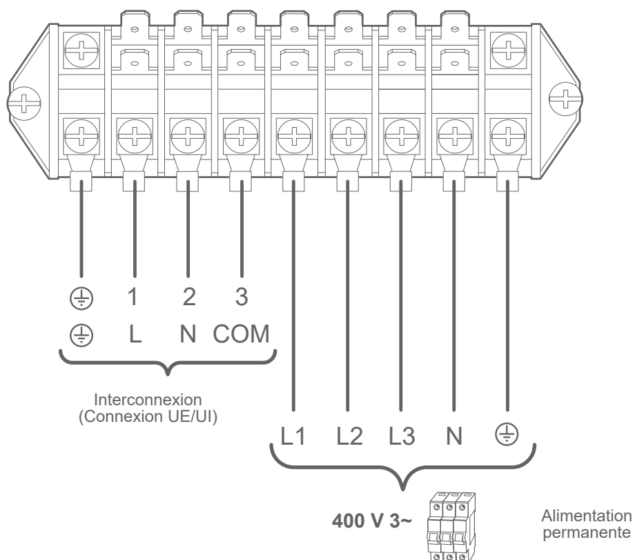
fig. 39 - Borniers de raccordement électrique coté unité extérieure
