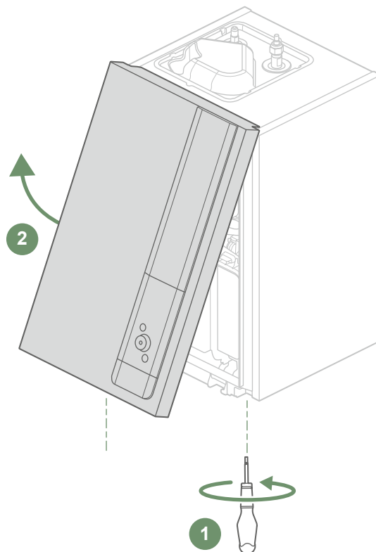
fig. 19 - Ouverture de la façade
