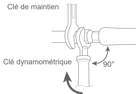
fig. 29 - Couples de serrage
