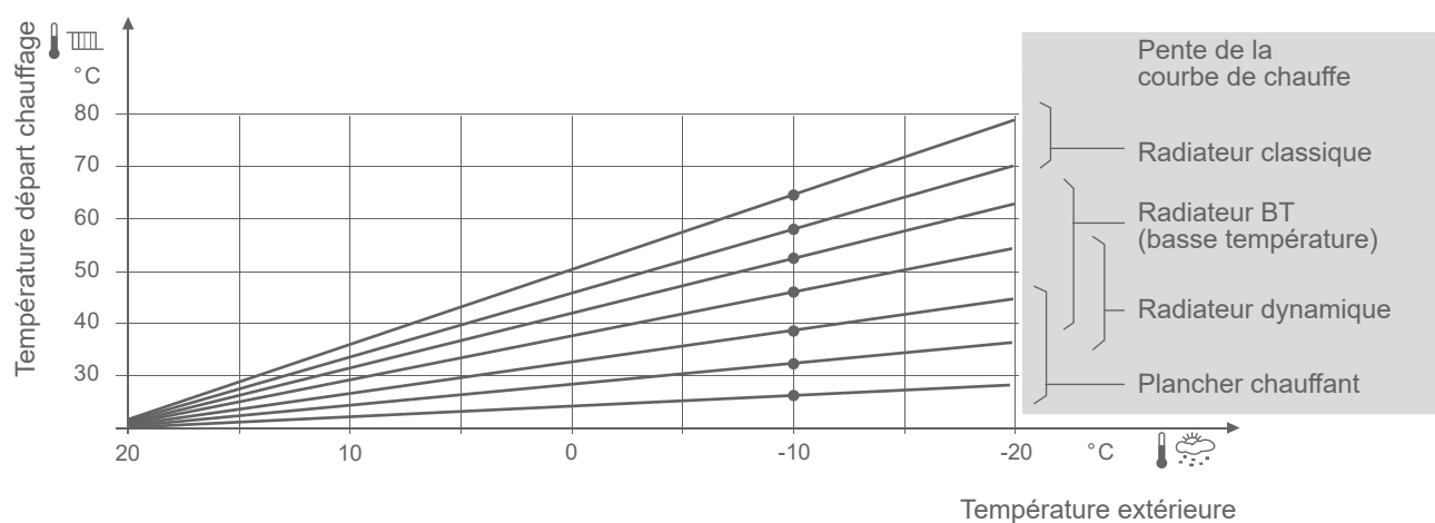
fig. 41 - Pente de la courbe de chauffe
