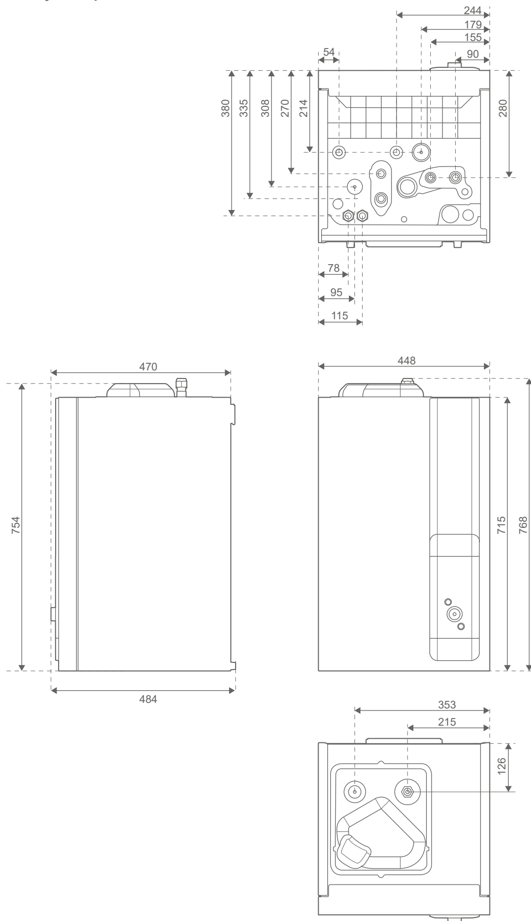
fig. 3 - Dimensions en mm
