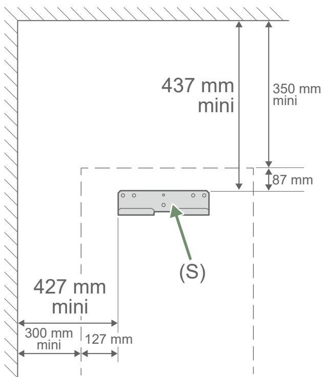
fig. 20 - Fixation murale
