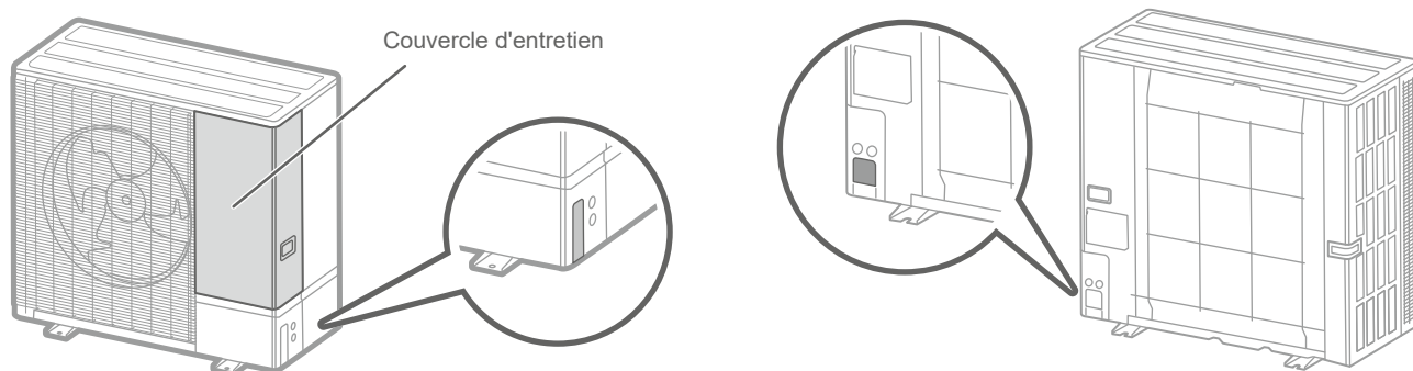
fig. 30 - Ouverture des trous prédécoupés
