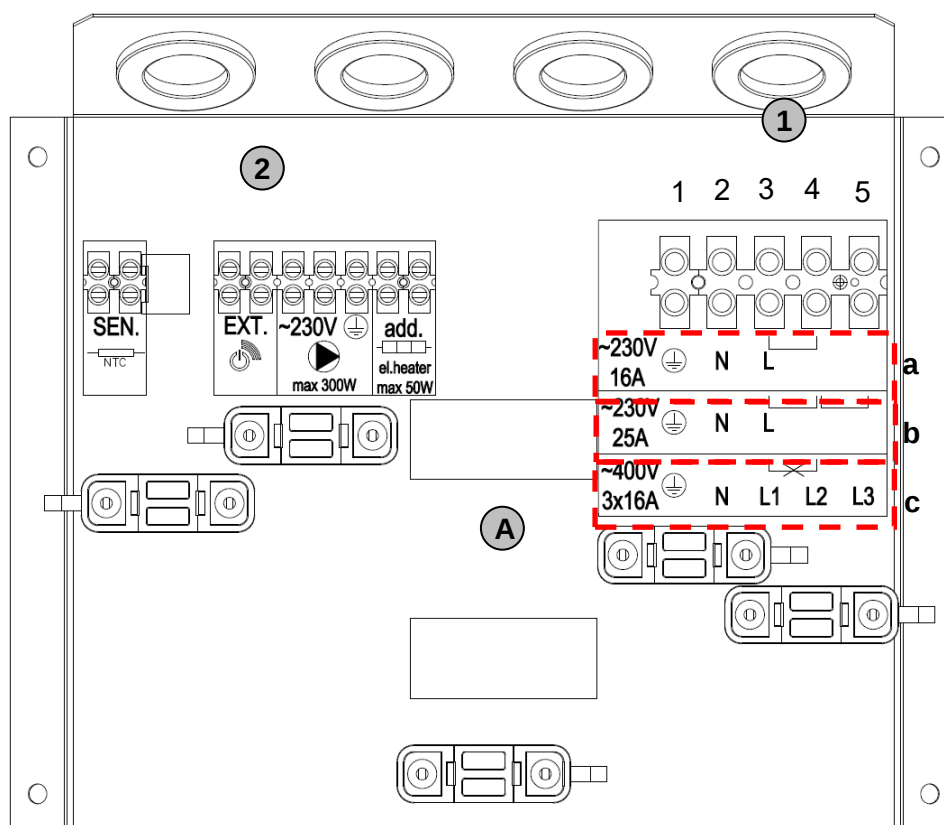
Fig. 7: Bornes électriques
