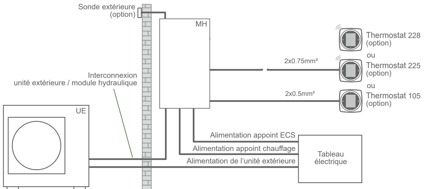
fig. 39 - Schéma d'ensemble des raccordements électriques pour une installation simple (1 circuit de chauffe)
