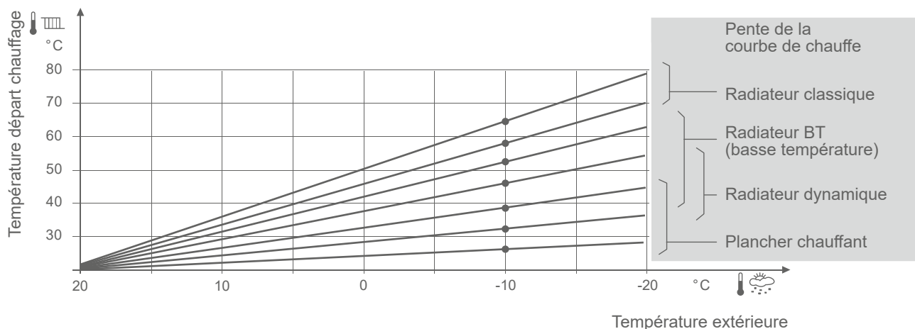
fig. 44 - Pente de la courbe de chauffe
