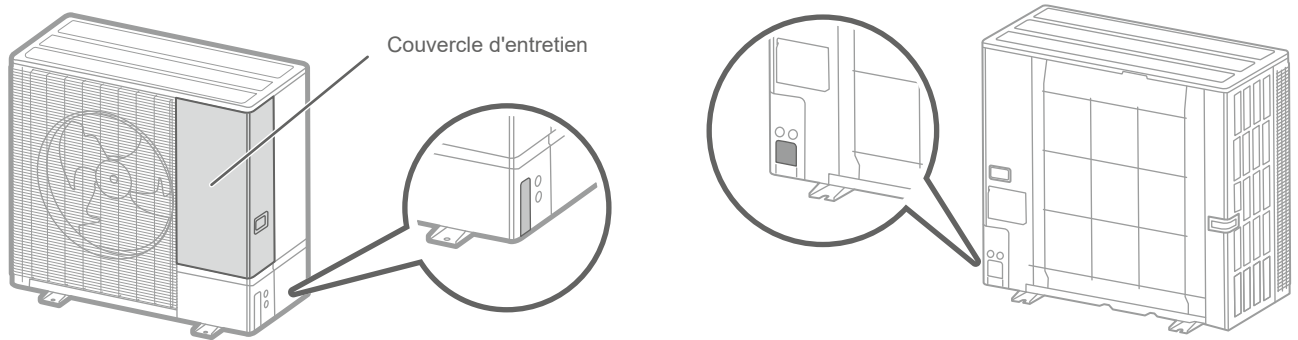
fig. 31 - Ouverture des trous prédécoupés
