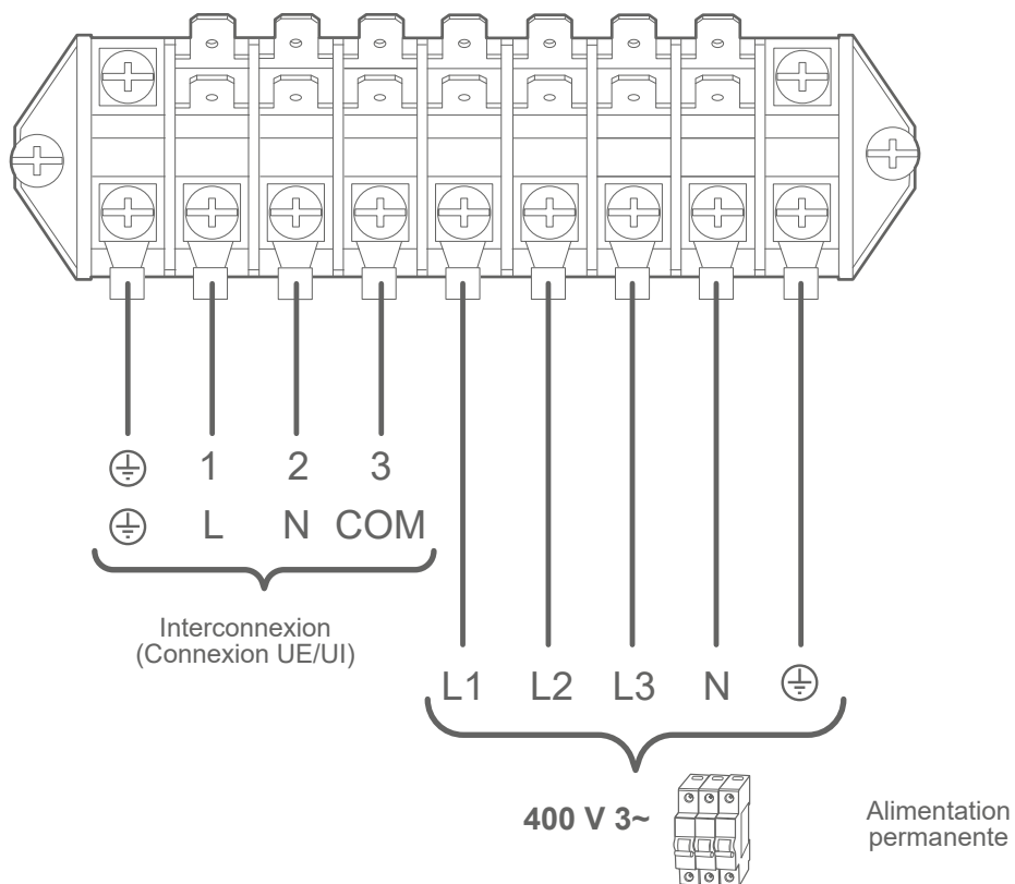
fig. 42 - Borniers de raccordement électrique coté unité extérieure
